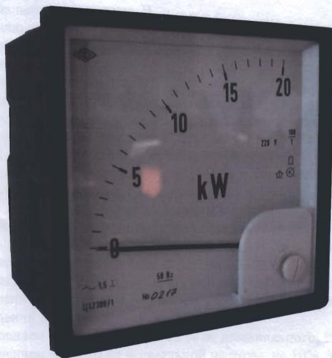
Рисунок 1 – Фотография ваттметра Ц42308/1
